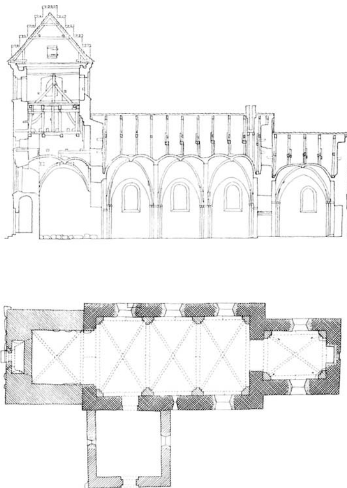
Fig. 3. Vejlbj. Længdesnit og plan 1: 300. Målt af Aksel Skov 1940 og elever fra Arkitektskolen i Århus 1975, tegnet med supplementer af KdeFL 1977. —Longitudinal section and ground-plan 1:300.
